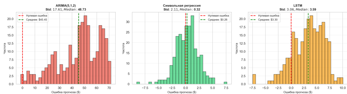
Рис. 7: Анализ ошибок прогнозирования
