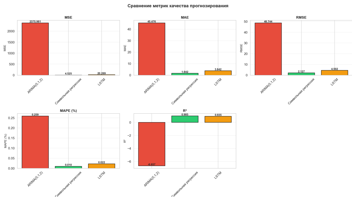
Рис. 8: Сравнение метрик качества
