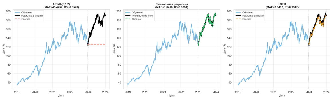
Рис. 6: Индивидуальные графики прогнозов для каждой модели
