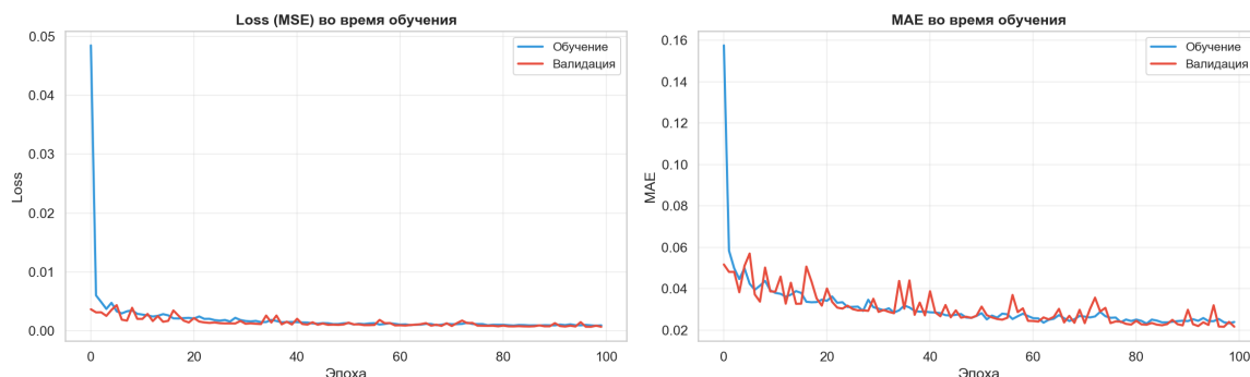
Рис. 4: История обучения LSTM: Loss (MSE) и MAE
