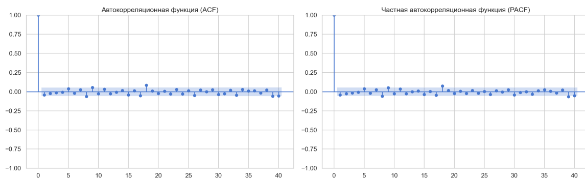
Рис. 3: ACF и PACF графики для выбора параметров ARIMA
